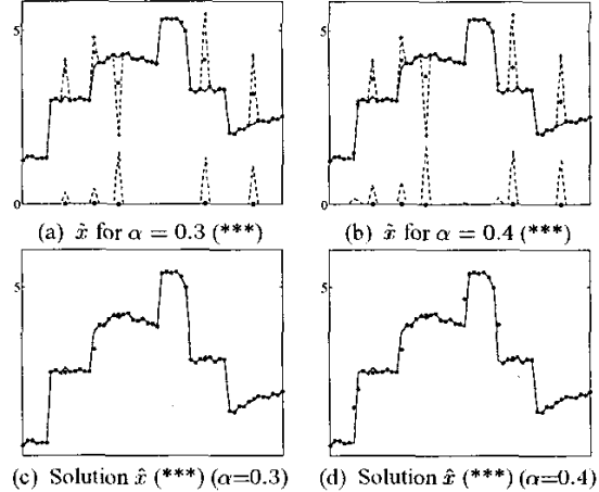
Fig. 1. Original (—), Data (---), Outliers in y (o), Residual |\hat{x} - y| (-.-).
